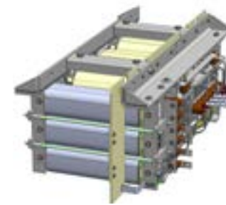
Tragrahmen Unterfluranwendung mit Drossel
