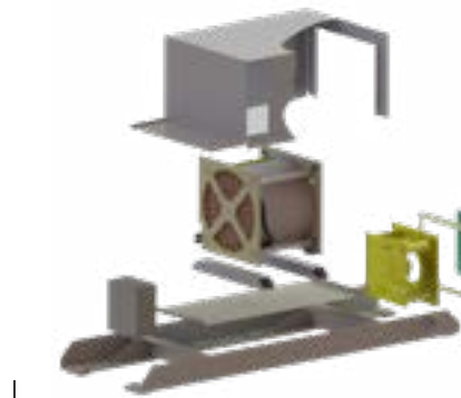
Explosionsgrafik Tragrahmen
